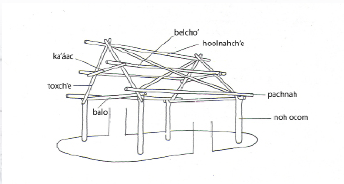
Fig. 3. Tectónica de la casa maya con los nombres de sus componentes estructurales Fuente: Basado en Villers et al., 1981 y mmodificada por el autor
